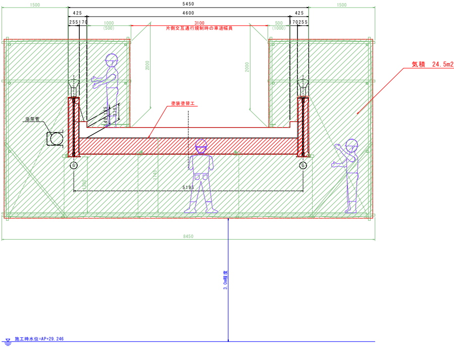
断面図 S=1:30
